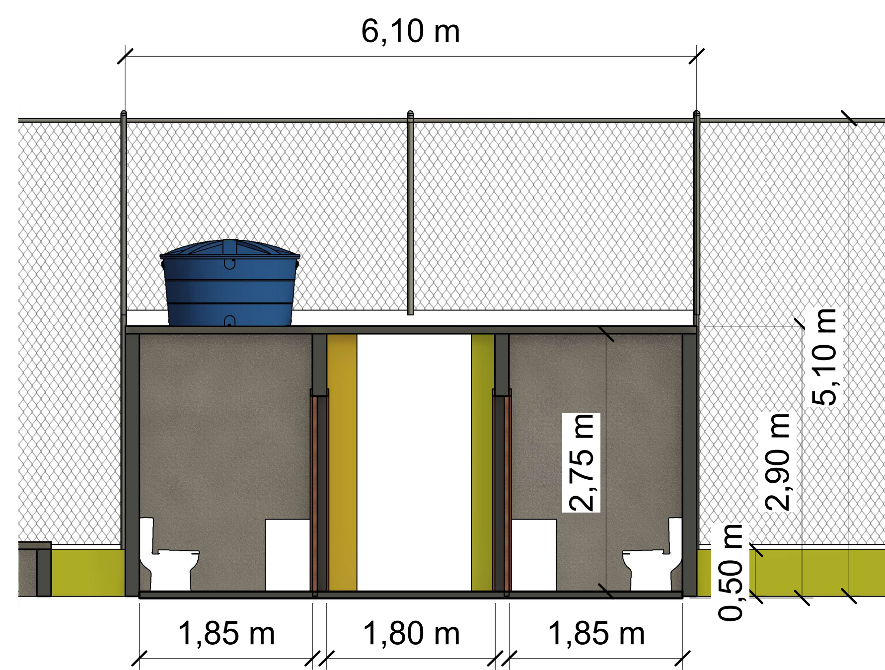
3 Corte 11 1 : 50
